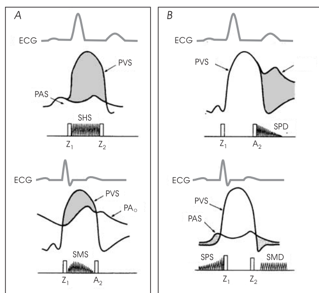
FIGURA 227-4 A. Reprezentare schematică a electrocardiogramei (ECG), presiunii aortice ( PA_0 ), presiunii în VS (PVS) și a presiunii în AS (PAS). Zonele hașurate reprezintă gradientul presional transvalvular în sistolă. SHS = suflu holosistolic; SMS = suflu mezosistolic. B. Reprezentare grafică a ECG, PA_0 , PVS și PAS cu zone hașurate indicând gradientul presional transvalvular în diastolă. SPD = suflu protodiastolic; SPS = suflu presistolic; SMD = suflu mezodiastolic.
